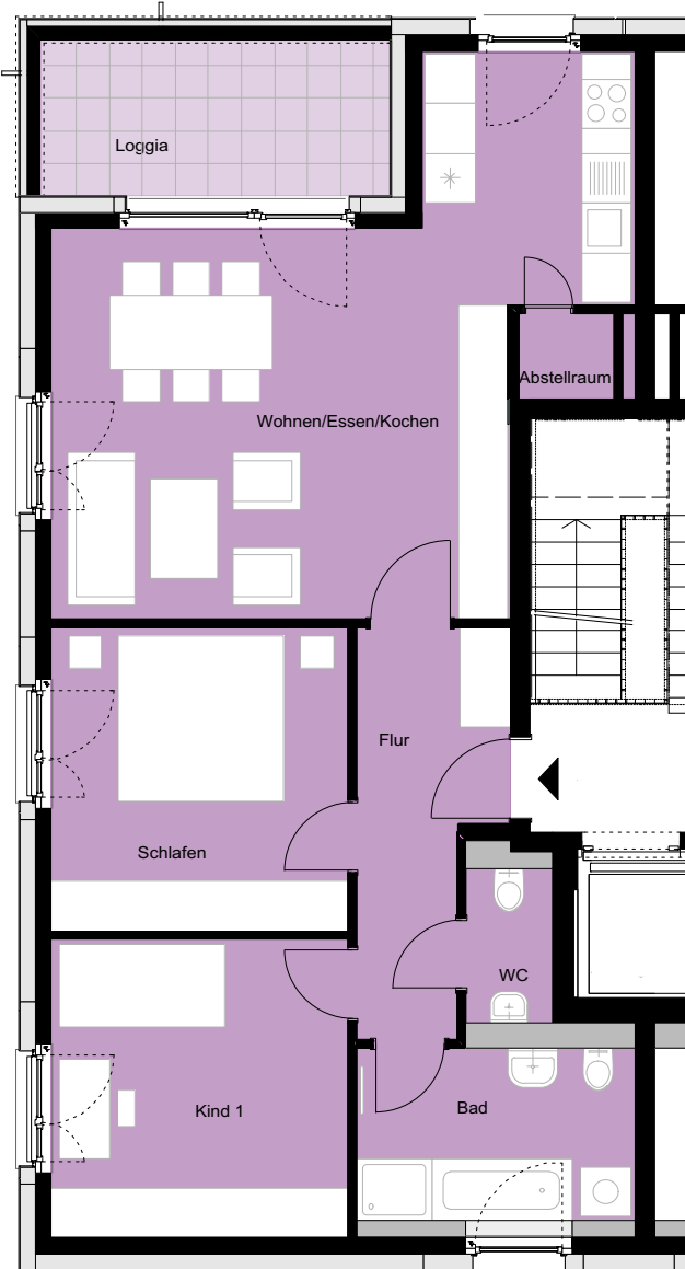
Grundriss M 1:100
