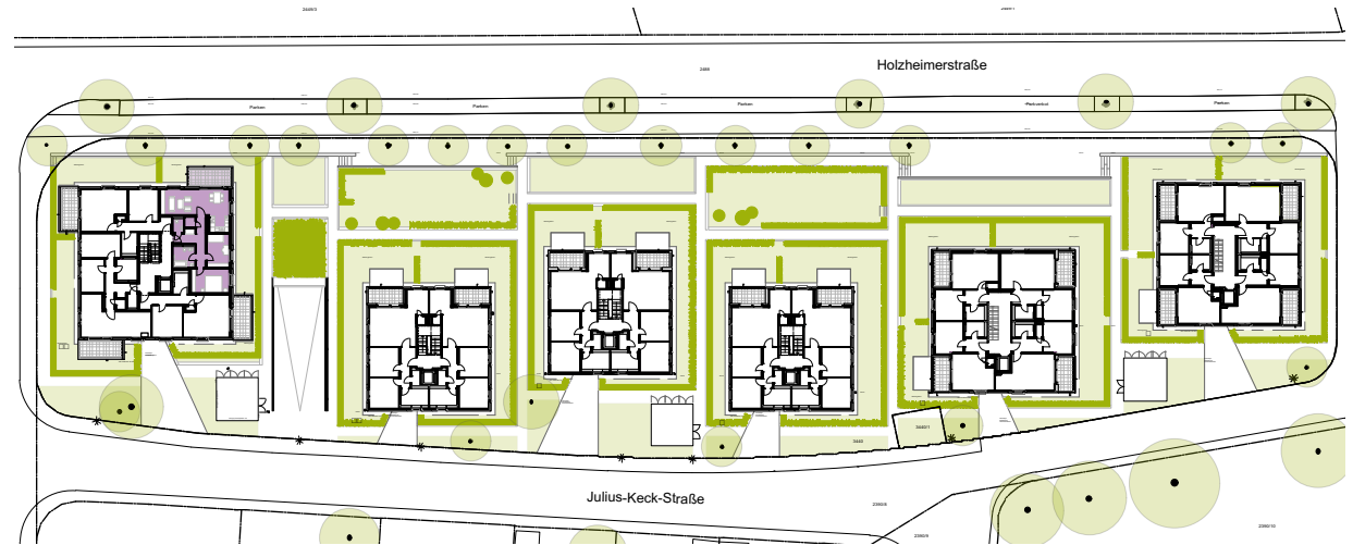
Übersicht M 1:1000
